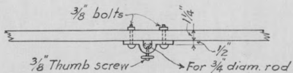
Plan.
