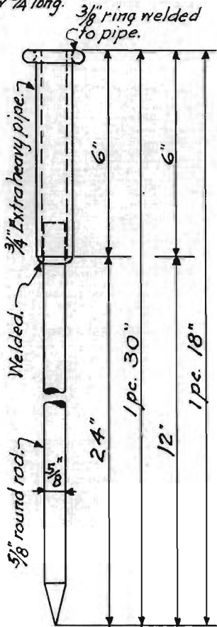
FLAG HOLDER STAKES. Scale: 3" = 1'-0"
