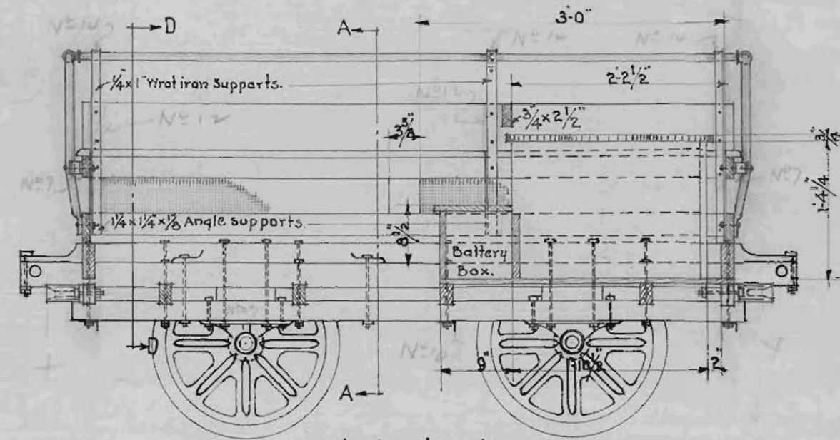
Longitudinal Section-B-B.
