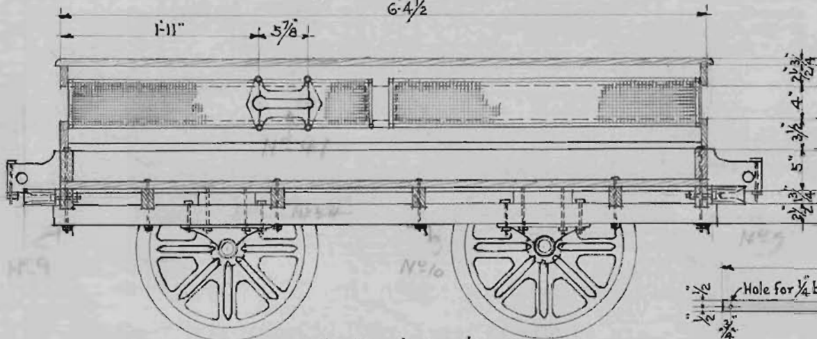
Longitudinal Section.C-C.
